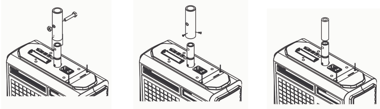
Рисунок 1.10 – Порядок монтажа верхних кронштейнов
